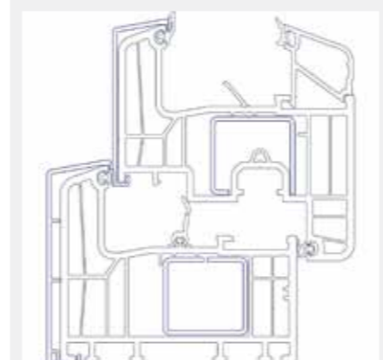
WIES Eforte plus mit Alu-Vorsatzschale
